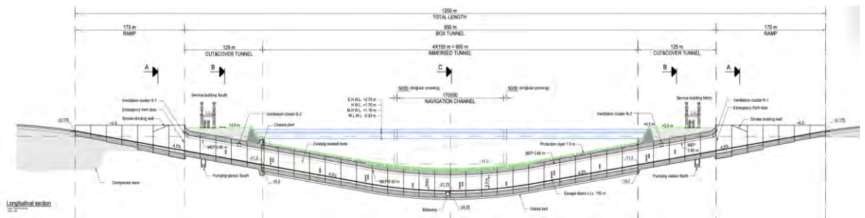
Figure Longitudinal section
